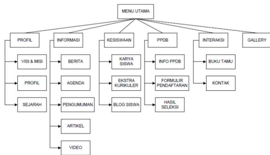
Gambar 4. Struktur Menu
