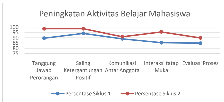
Gambar 1. Grafik Peningkatan Aktivitas Belajar Mahasiswa
