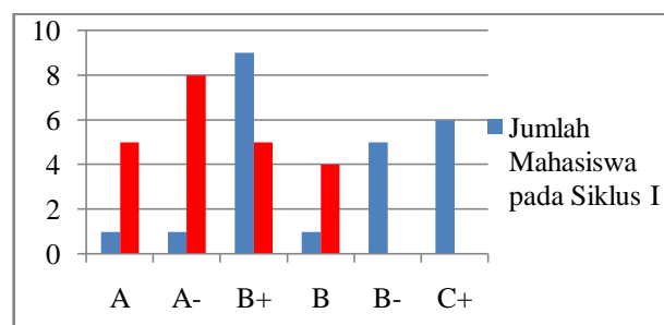
Gambar 2. Grafik Peningkatan Hasil Belajar Kognitif Mahasiswa
