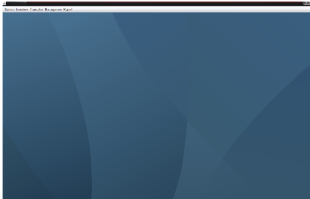
Gambar 3. 1 Halaman Utama
